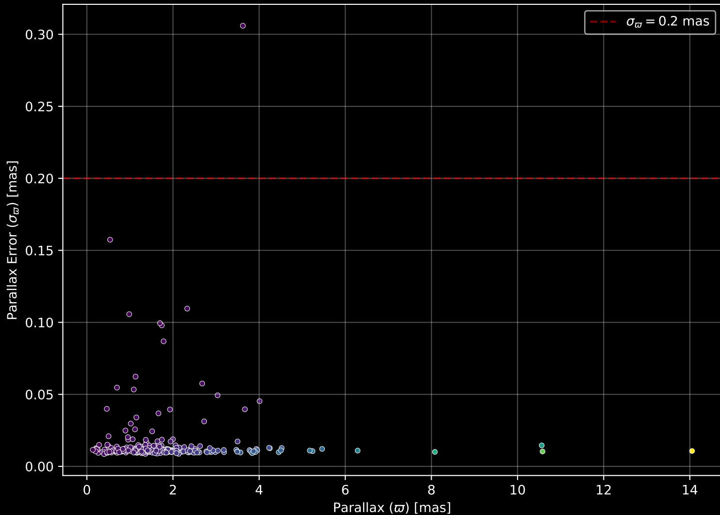
GALAH DR4 Field: [129] Parallax Quality (n= 289)
