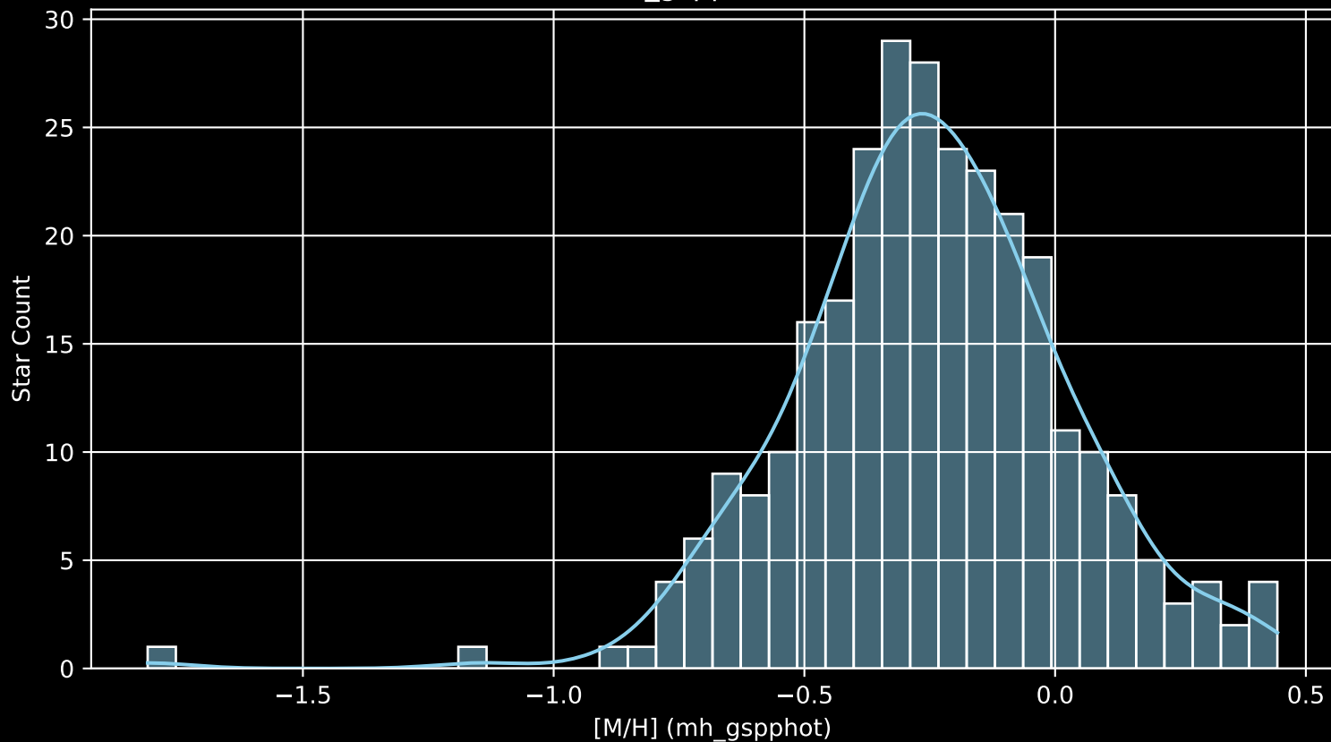
GALAH DR4 Field: [129] [M/H] (mh_gspphot) (n= 289)
