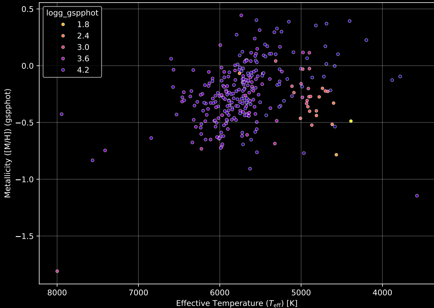
GALAH DR4 Field: [129] Stellar Population Parameters (n= 289)
