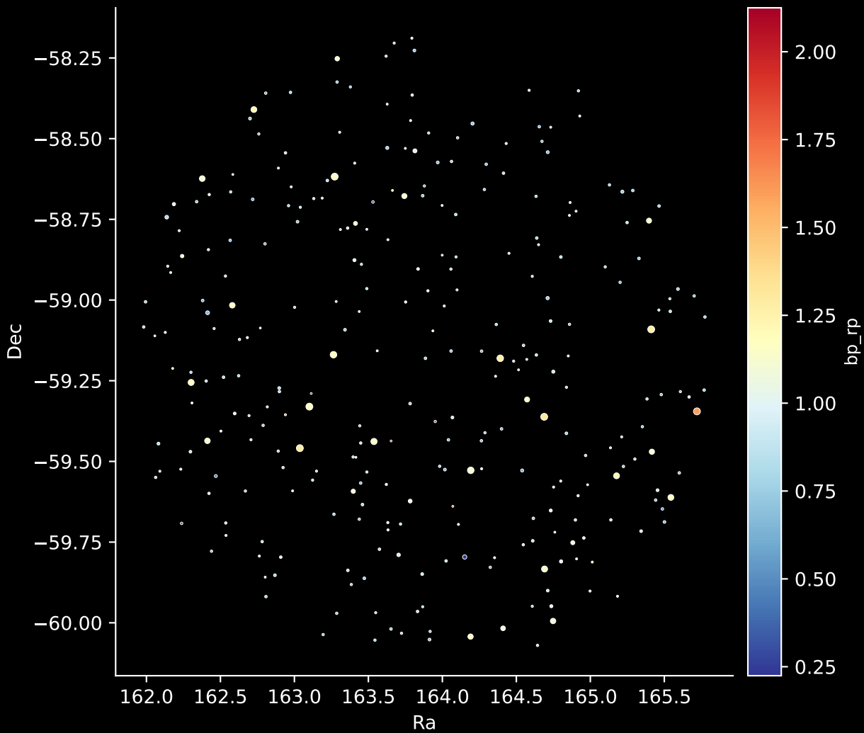
GALAH DR4 Field: [129] Stars: 289
